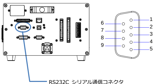
RS232C シリアル通信コネクタ
