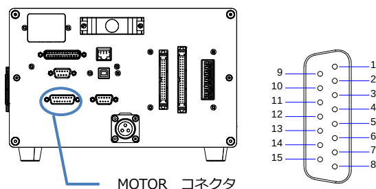
MOTOR コネクタ
